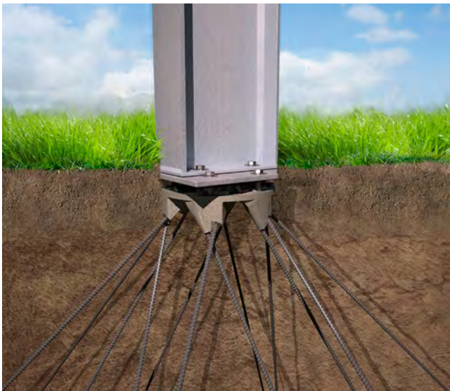
Abb. 60: Spinnanker mit Ankerplatte und Gewindestäben fundamentieren das Montagesystem im Boden © Spinnanker GmbH
