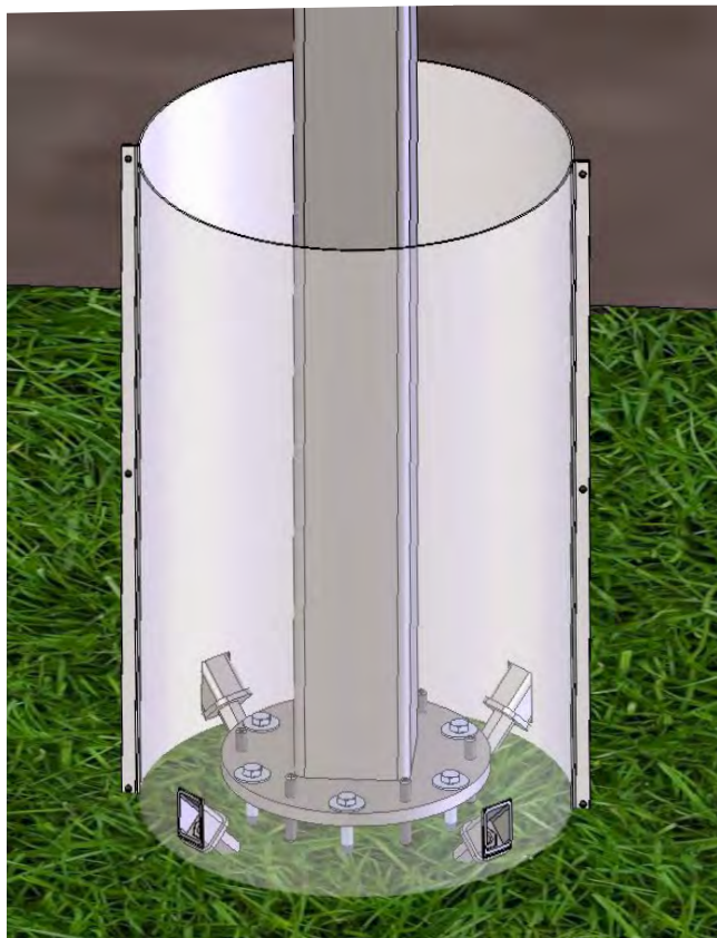
Abb. 38: Rammschutz der Aufständigung der Anlage in Heggelbach gegen mögliche Beschädigungen durch Landmaschinen © AGROSOLAR Europe GmbH
