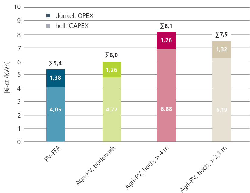
Abb. 48: Geschätzte Stromgestehungskosten unterteilt nach Investitionsausgaben (CAPEX) und Betriebskosten (OPEX) von PV-Freiflächenanlagen und Agri-PV im Vergleich © Fraunhofer ISE
