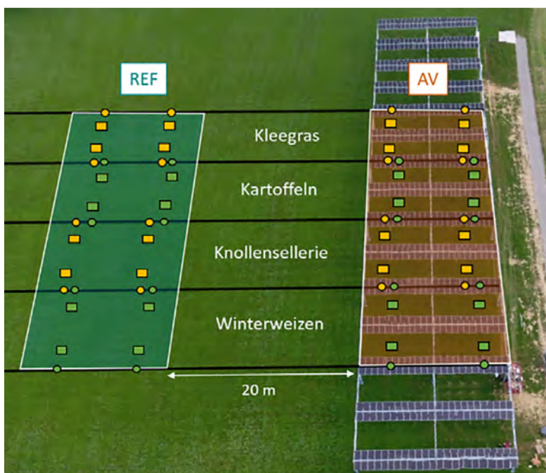
Abb. 36: Feldplan des Versuchsaufbaus 2017 mit Messstationen. Bereiche in denen Proben entnommen wurden, werden durch Kästchen, Positionen von Mikroklimastationen durch Kreise angezeigt © BayWa r.e., verändert durch Axel Weselek/Universität Hohenheim.
