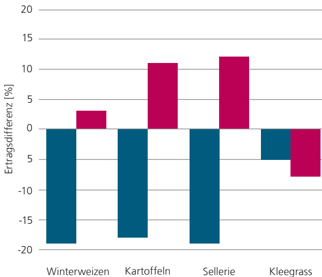
Abb. 37: Ertragsunterschiede der Kulturen unter Agri-PV gegenüber Referenzflächen 2017 (blau) und 2018 (rot) in Heggelbach (ohne Flächenverluste durch Stützen). Daten: Universität Hohenheim, © Fraunhofer ISE
