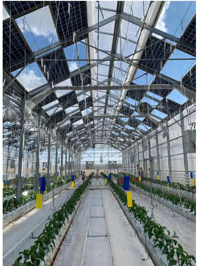
Abb. 34: PV-Gewächshaus © Fraunhofer ISE
