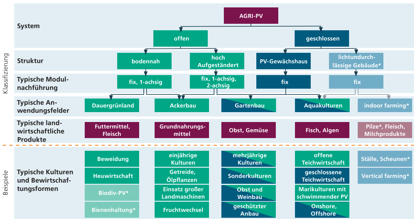
Abb. 9: Klassifizierung von Agri-PV-Systemen
