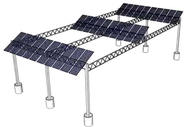
Abb. 61: Illustration verschiedener Anlagentypen mit Ost-West-, Süd- und Süd-Ost-Ausrichtung © Fraunhofer ISE
