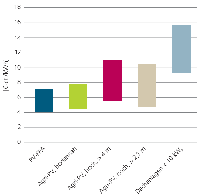
Abb. 49: Geschätzte Stromgestehungskosten (LCOE) für PV-Freiflächenanlagen und Agri-PV
